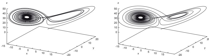
Abbildung 11.3: Numerisch berechnete Lösungstrajektorien für das Lorenz-System; links: korrektes Ergebnis; rechts: falsches Ergebnis
