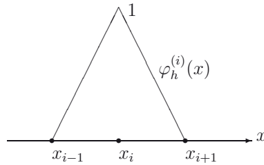
Abbildung 11.1: Lagrange-Basisfunktion linearer finiter Elemente
