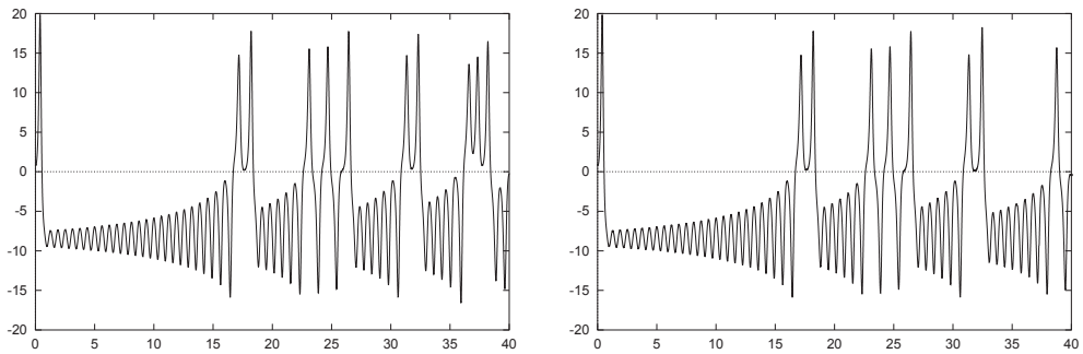
Abbildung A.1: Referenzlösung (x-Komponente) (links) und „falsche“ Lösung (x-Komponente) (rechts) auf dem Intervall I = [0, 40] berechnet mit dem adaptiven dG(1)-Verfahren mit \text{TOL} = 10^{-4} .
